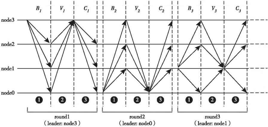
图1 Libra 的交易验证过程
